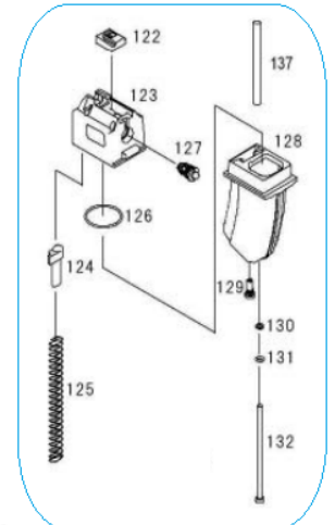
SHORT MAG
