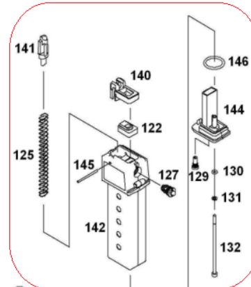
STANDARD MAG
